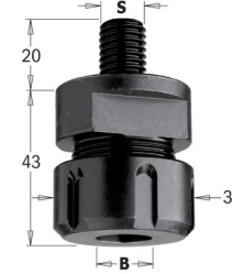
ER20 PENS MANDRENİ M14 ER20 CHUCK M14
